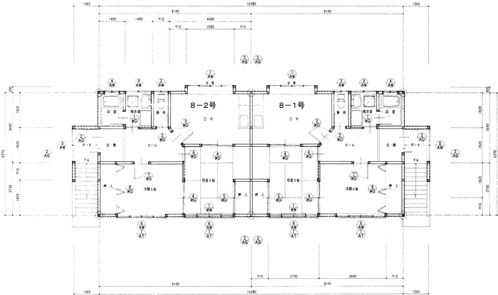
2階建具配置図 S=1:50
